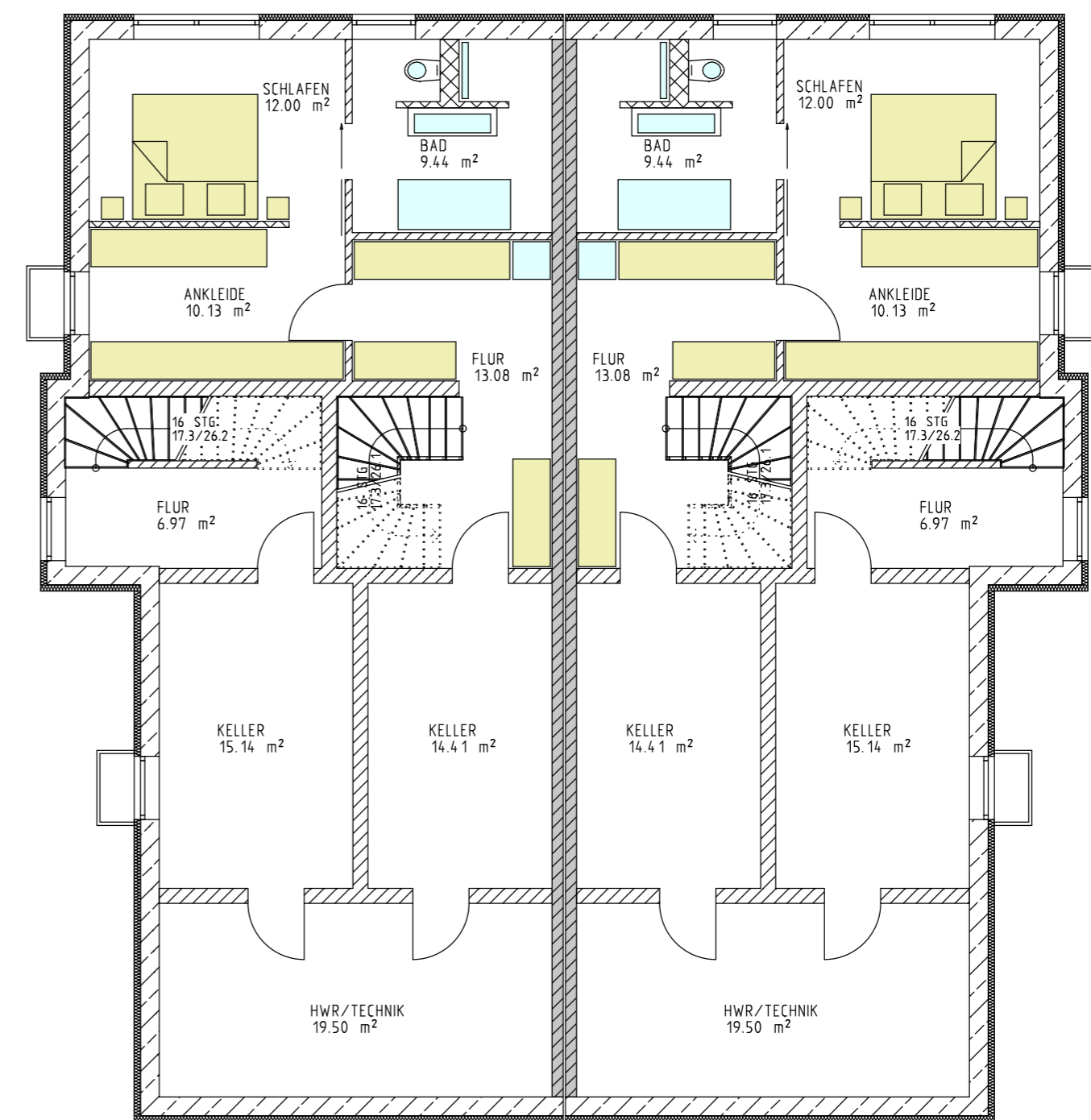
GRUNDRISS UNTERGESCHOSS
