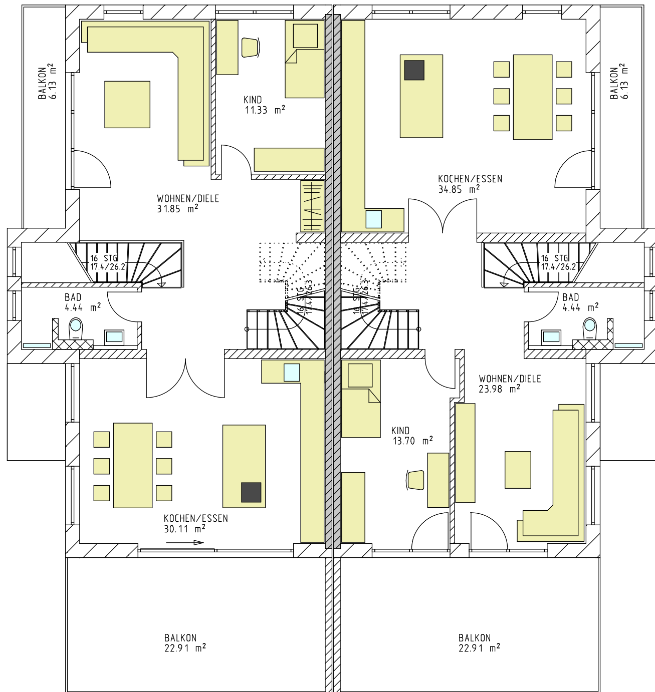
Maisonette-Wohnung OG+DG ca. 135 m 2
